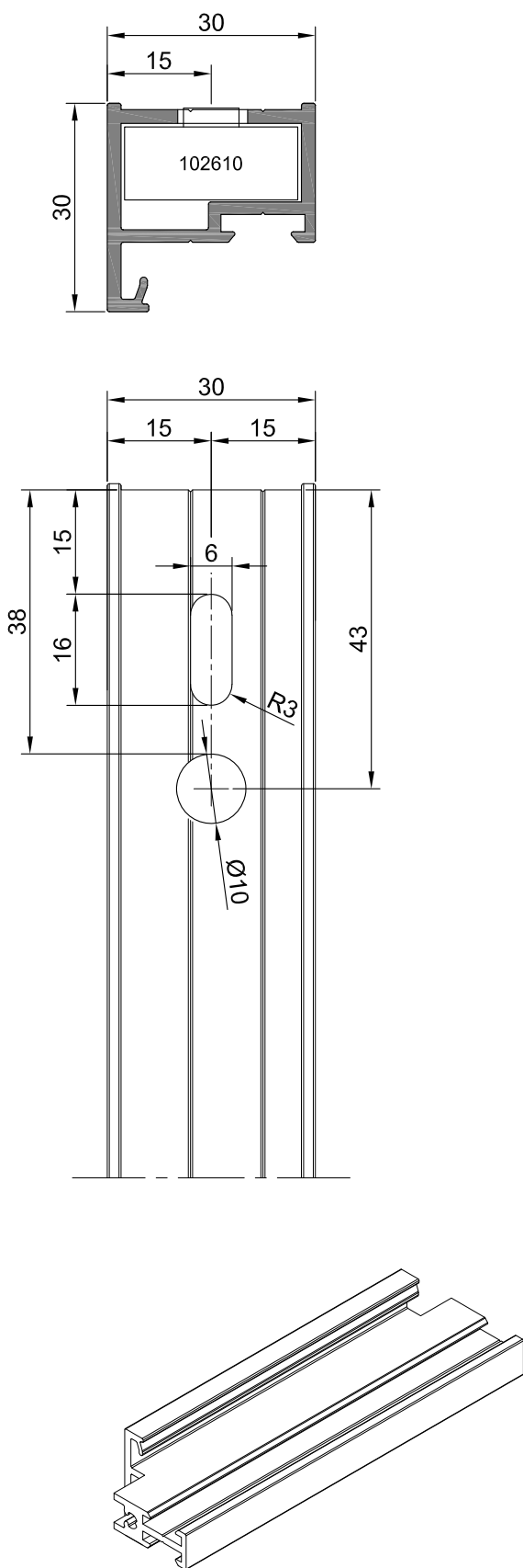
Mecanizado perfil 1S1250
