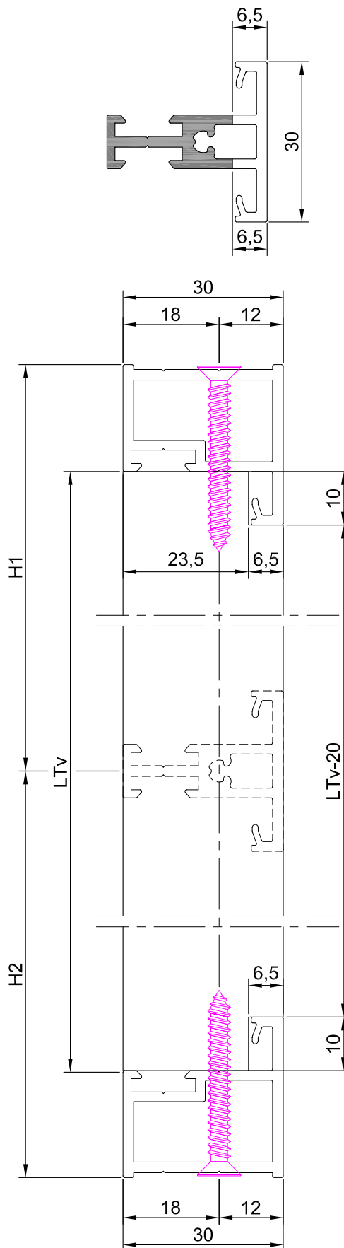
Fresado colocación 1S1300
