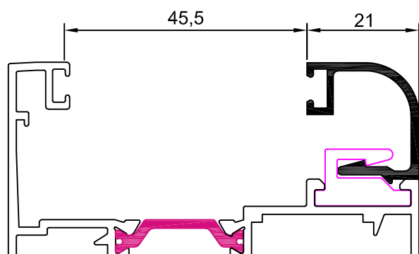
12003 junquillo 21 mm
