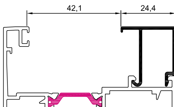
10006 junquillo 24,4 mm
