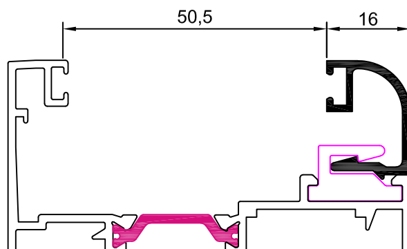
12002 junquillo 16 mm
