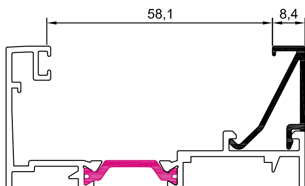
10001 junquillo 8,4 mm
