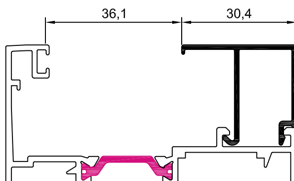
10008 junquillo 30,4 mm
