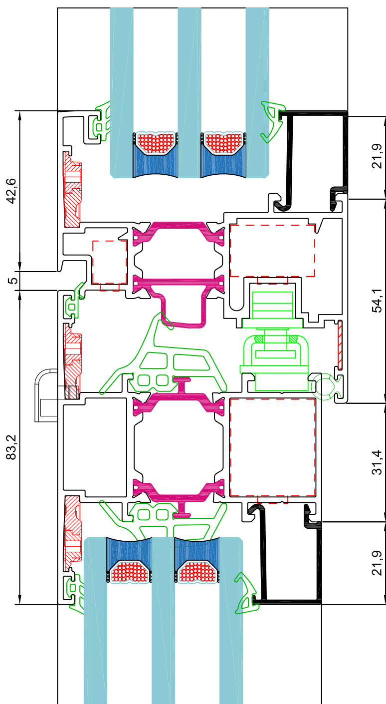
sección 6
