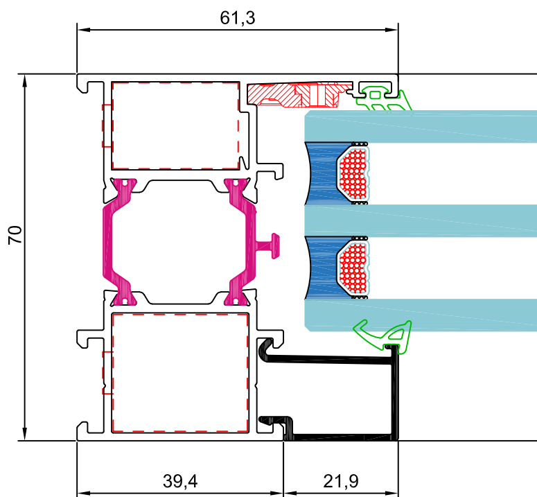
sección 1
