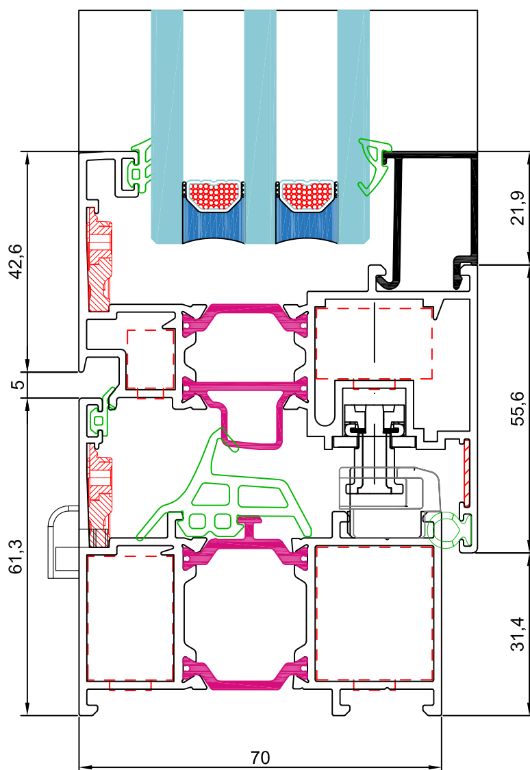
sección 4
