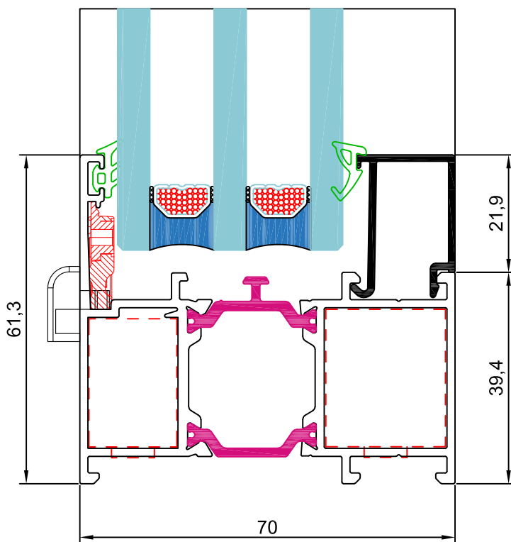
sección 2
