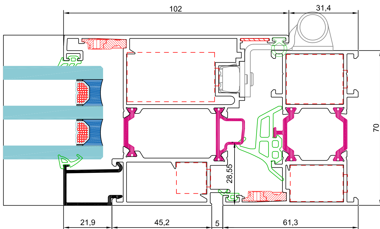
sección 10
