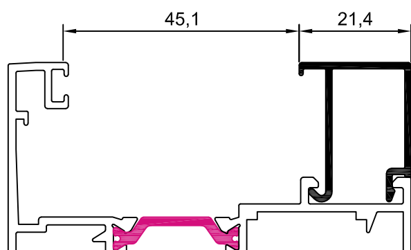
10005 junquillo 21,4 mm
