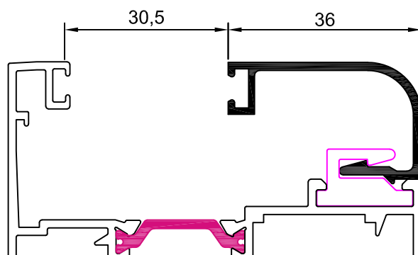
12006 junquillo 36 mm
