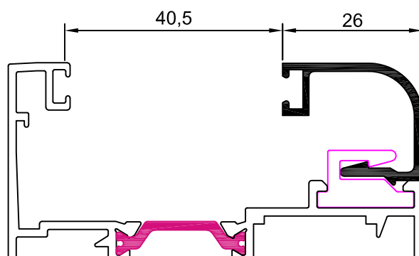
12004 junquillo 26 mm
