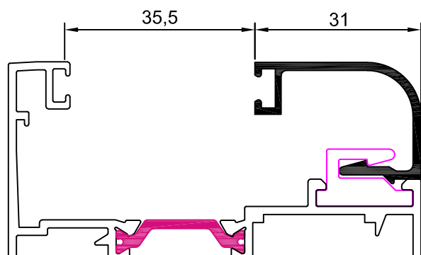
12005 junquillo 31 mm
