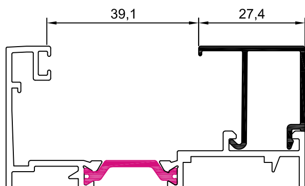
10007 junquillo 27,4 mm
