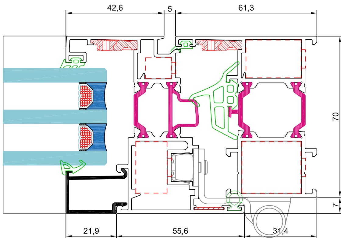
sección 3
