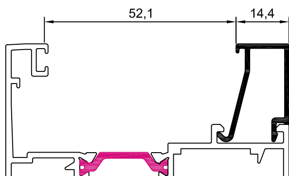
10003 junquillo 14,4 mm
