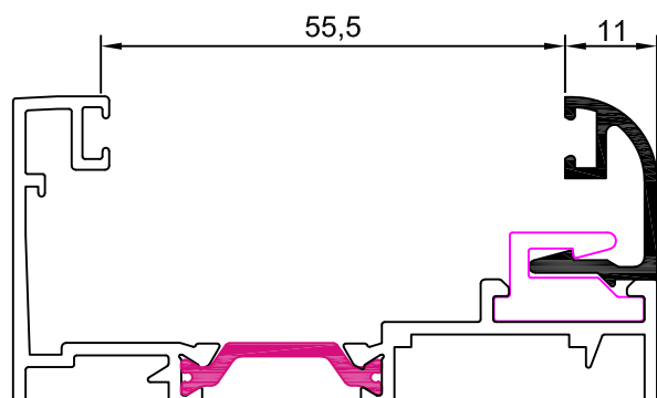
12001 junquillo 11 mm
