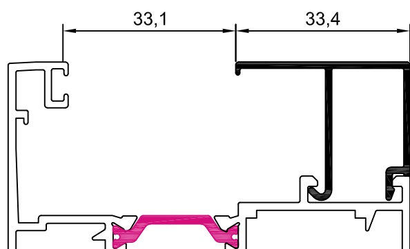
10009 junquillo 33,4 mm
