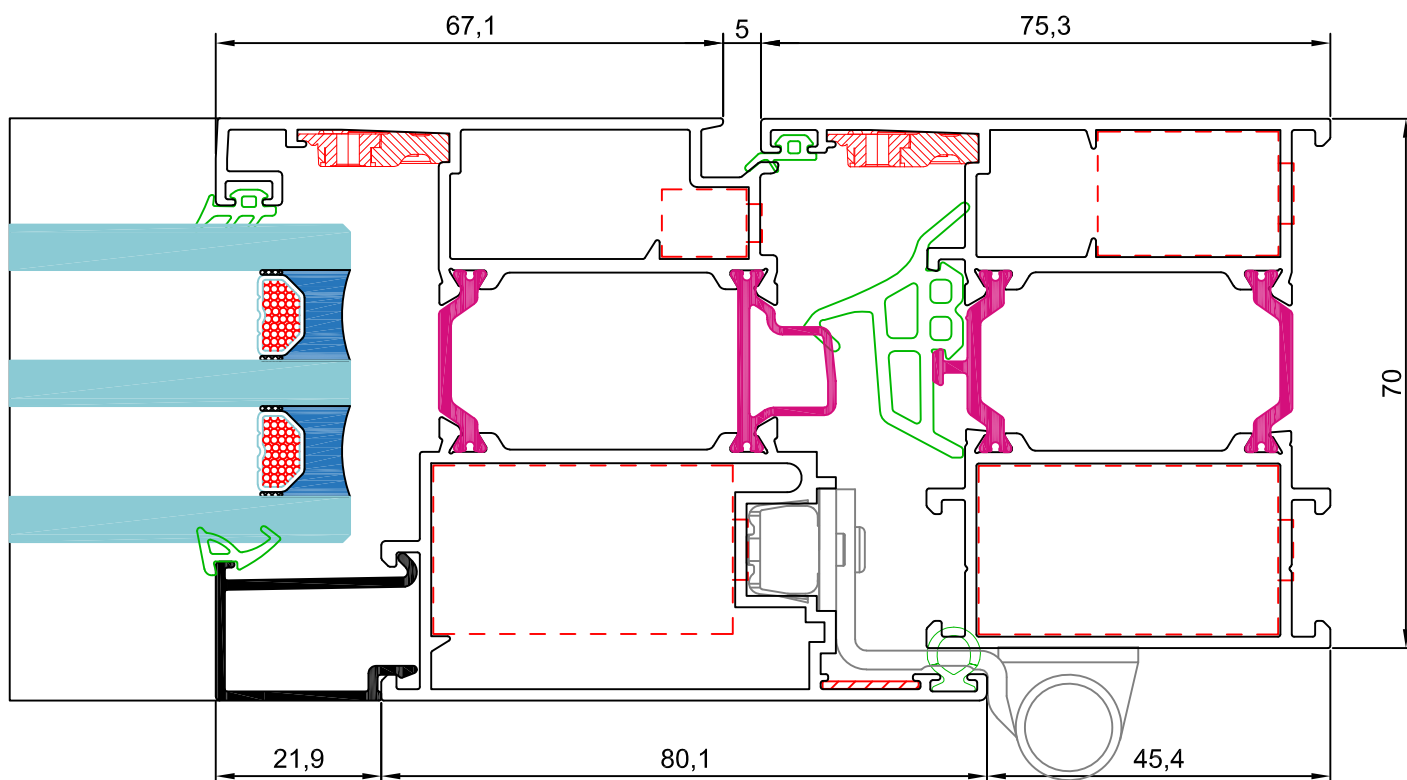
sección 7
