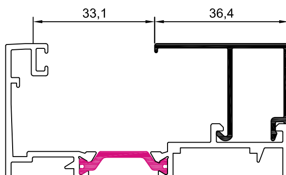
10010 junquillo 36,4 mm
