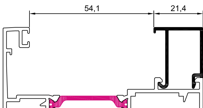
10005 junquillo 21,4 mm
