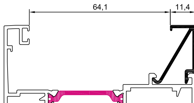
10002 junquillo 11,4 mm
