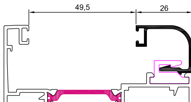
12004 junquillo 26 mm
