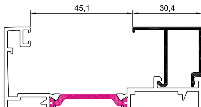
10008 junquillo 30,4 mm
