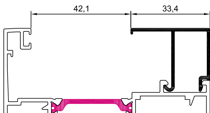
10009 junquillo 33,4 mm
