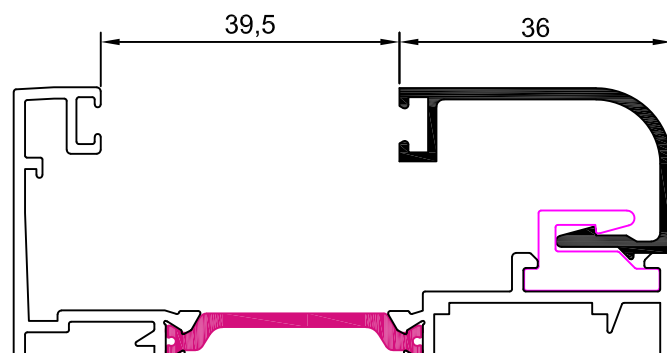
12006 junquillo 36 mm
