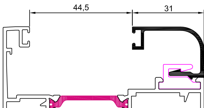
12005 junquillo 31 mm
