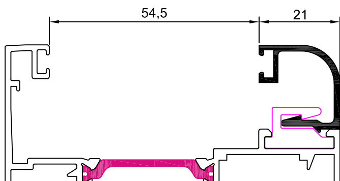
12003 junquillo 21 mm
