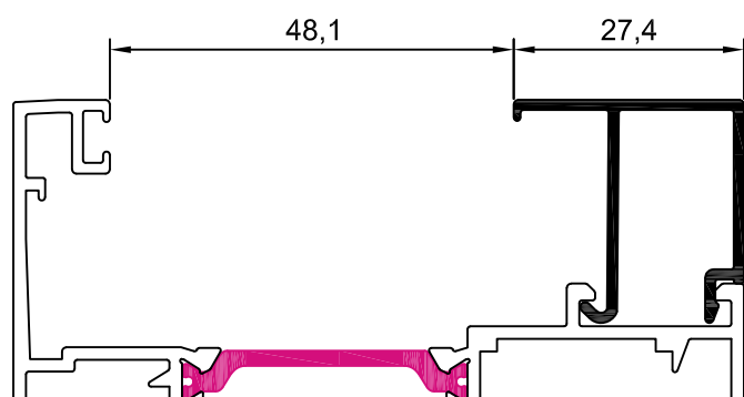
10007 junquillo 27,4 mm
