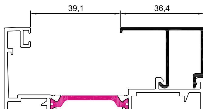
10010 junquillo 36,4 mm
