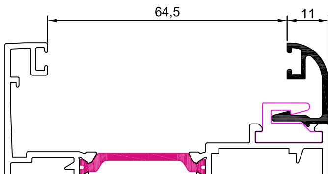
12001 junquillo 11 mm
