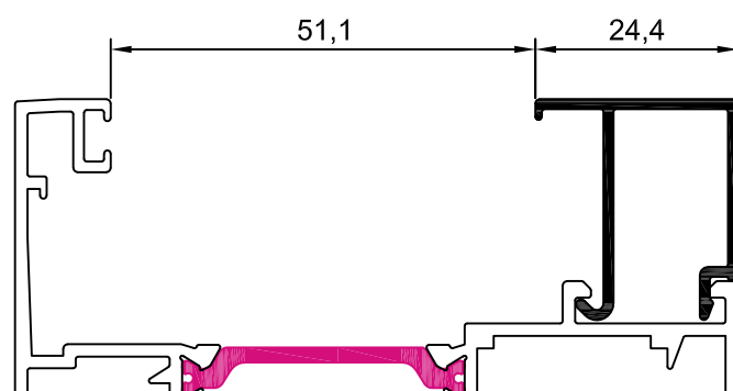
10006 junquillo 24,4 mm
