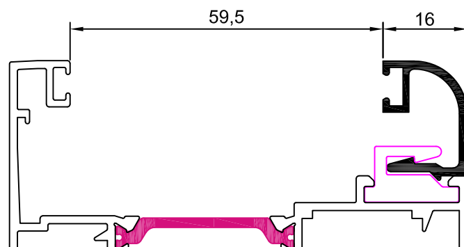
12002 junquillo 16 mm
