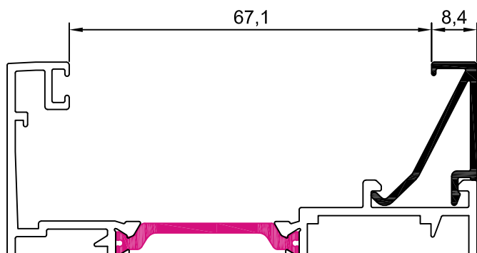
10001 junquillo 8,4 mm
