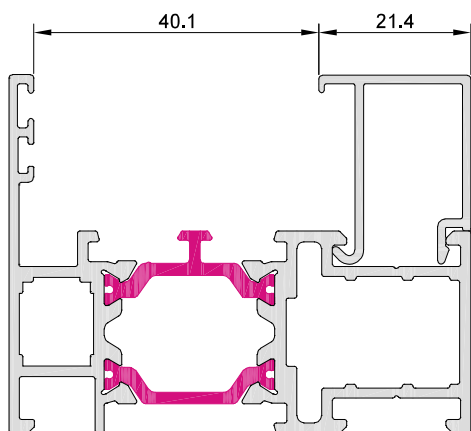
10005 junquillo 21,4 mm
