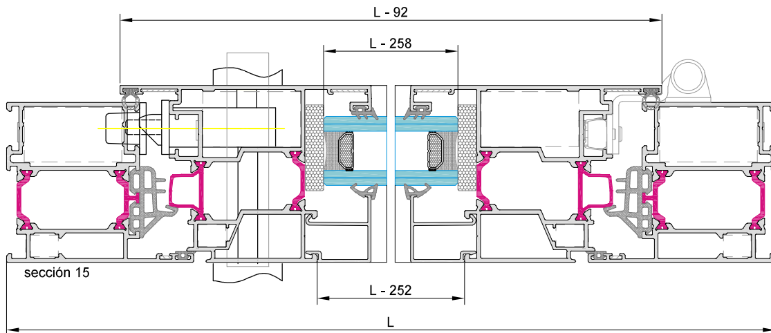
Escala Sección 1:2
