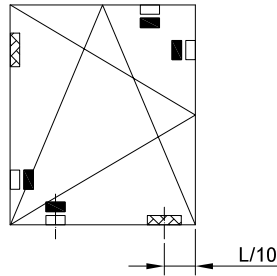
BASTIDOR OSCILOBATIENTE
