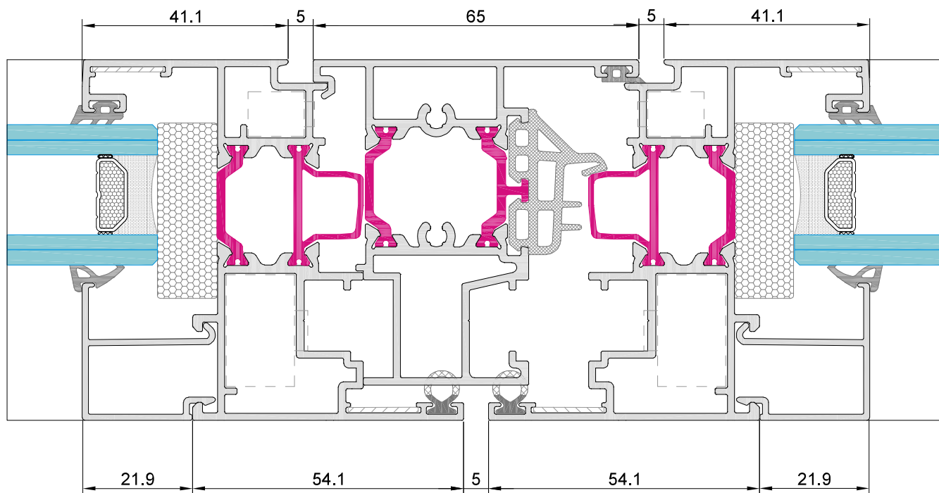
sección 7
