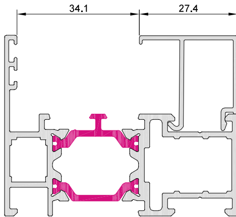
10007 junquillo 27,4 mm
