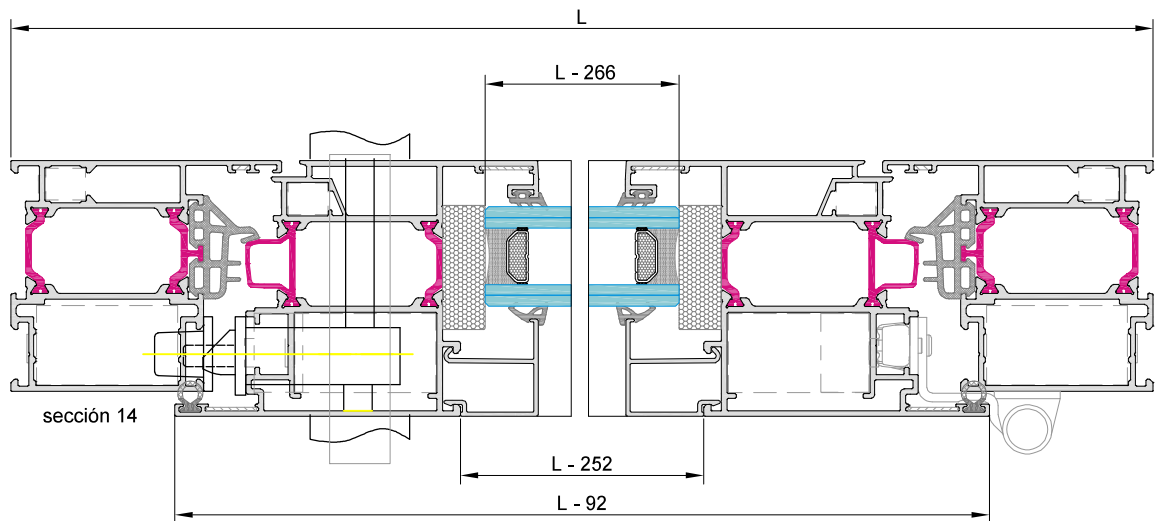
Escala Sección 1:2
