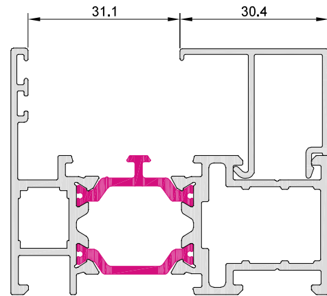
10008 junquillo 30,4 mm
