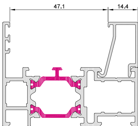
10003 junquillo 14,4 mm
