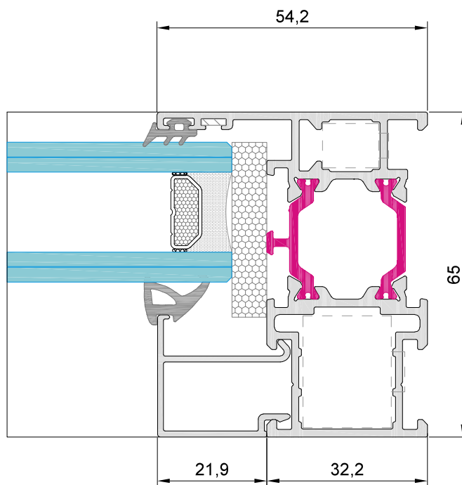
sección 1
