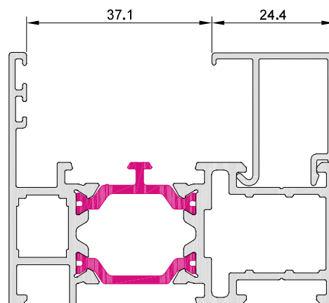
10006 junquillo 24,4 mm
