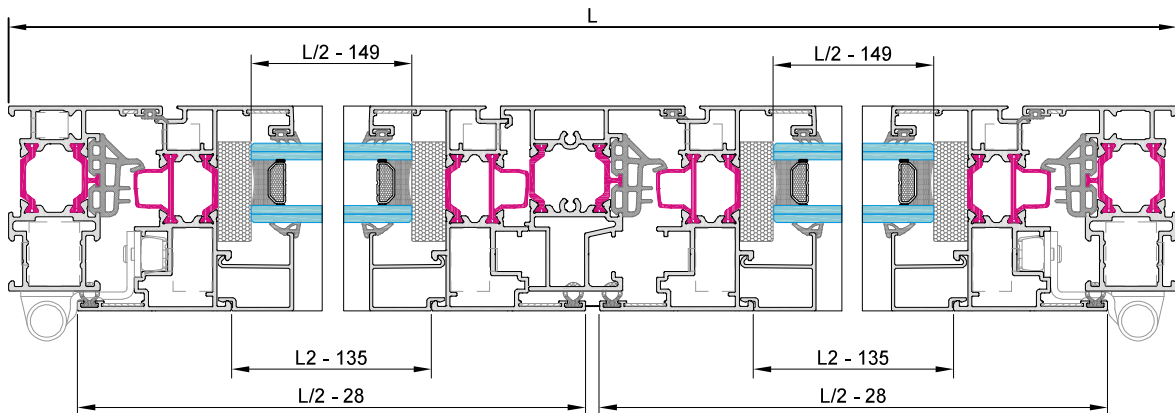
Escala Sección 1:4
