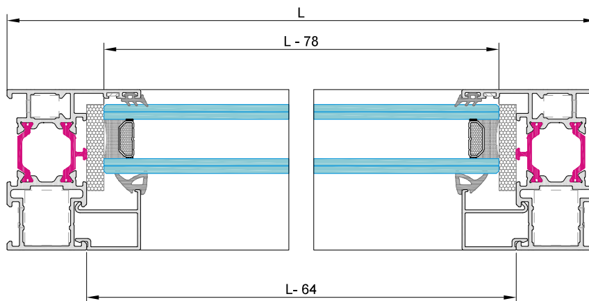
Escala Sección 1:2
