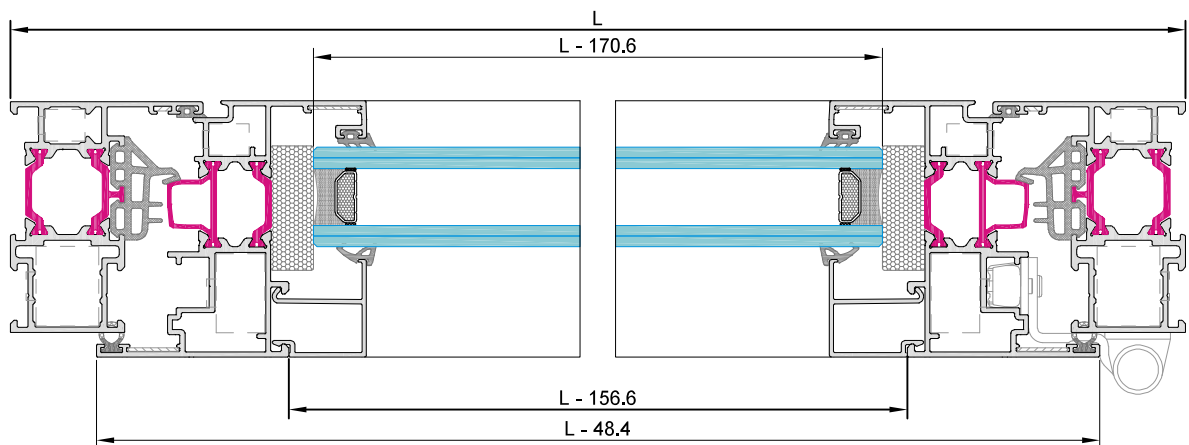
Escala Sección 1:2
