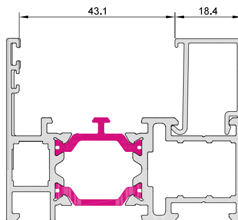
10004 junquillo 18,4 mm
