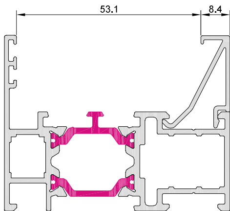
10001 junquillo 8,4 mm
