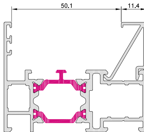
10002 junquillo 11,4 mm
