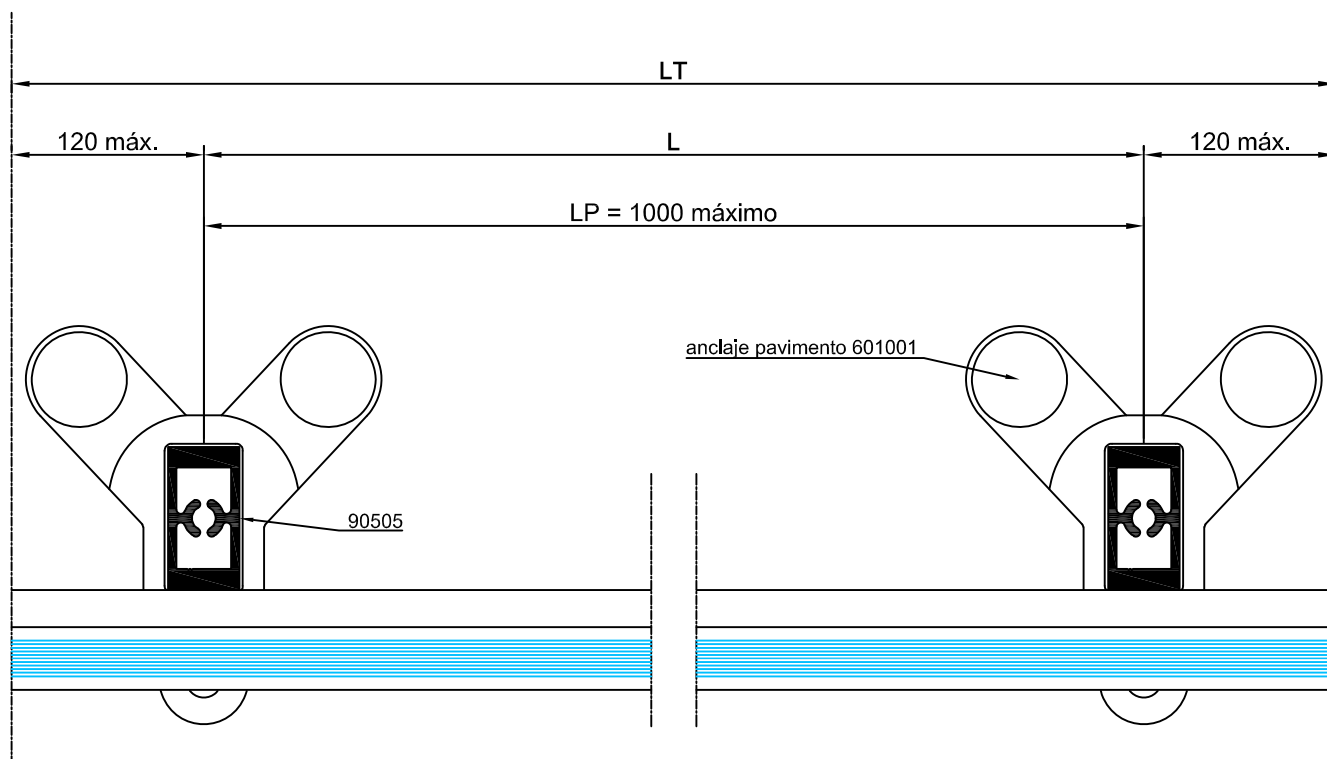
Sección 2
