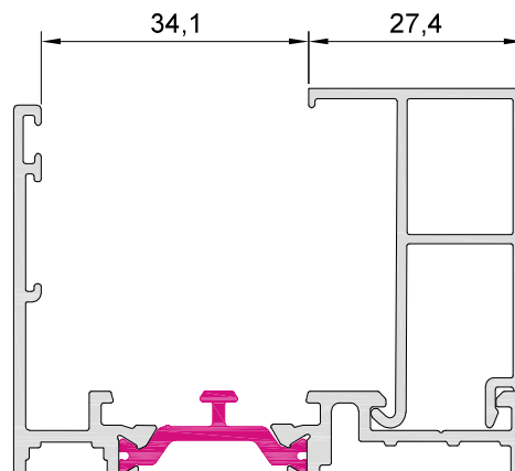
60537 junquillo 27,4 mm
