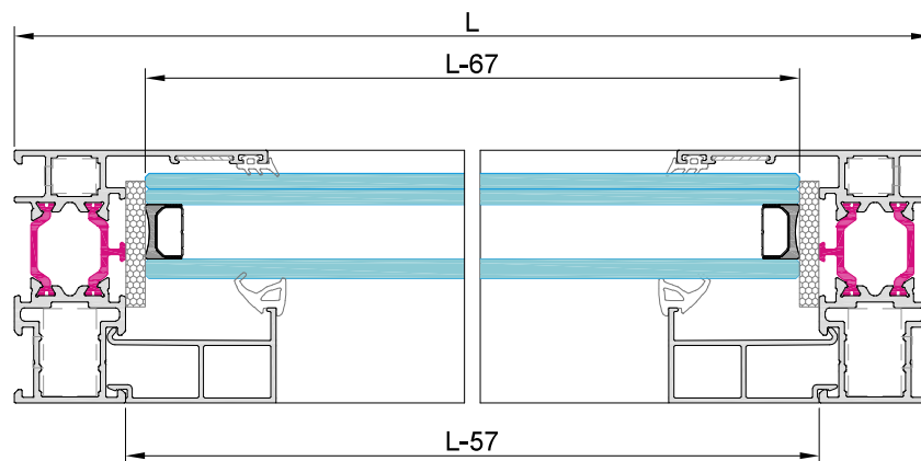
Escala Sección 1:2
