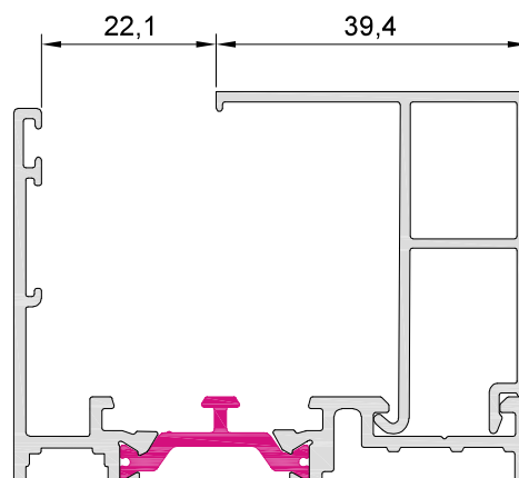
60542 junquillo 39,4 mm
