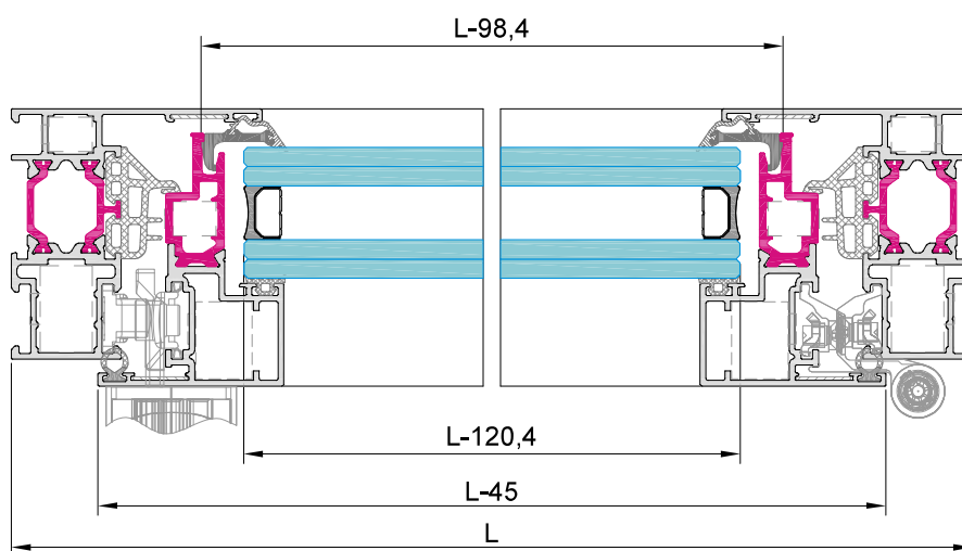
Escala Sección 1:2
