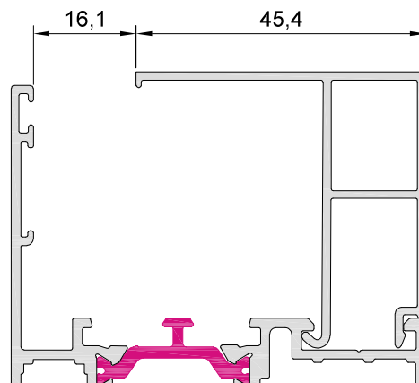
60544 junquillo 45,4 mm
