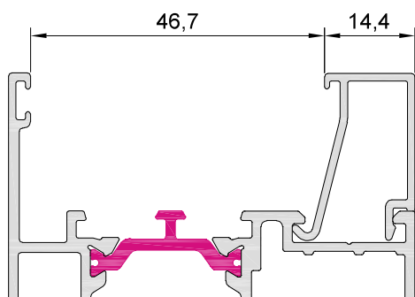
10003 junquillo 14,4 mm
