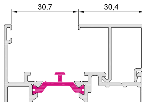
10008 junquillo 30,4 mm
