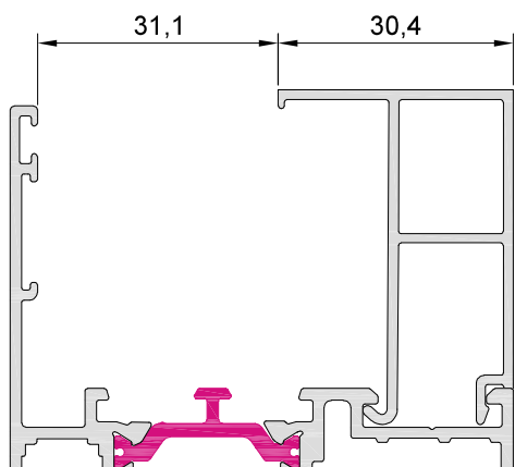
60538 junquillo 30,4 mm
