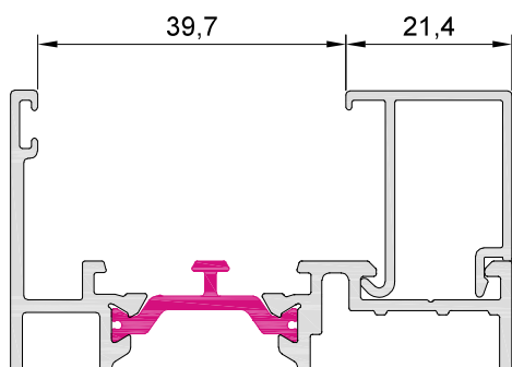
10005 junquillo 21,4 mm
