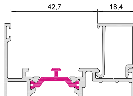
10004 junquillo 18,4 mm
