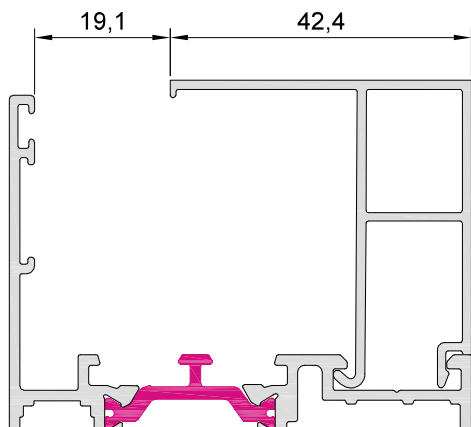
60543 junquillo 42,4 mm
