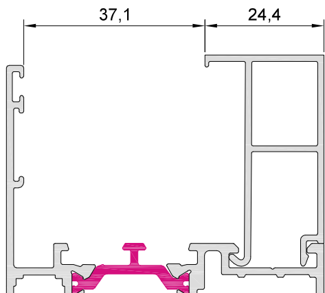
60536 junquillo 24,4 mm
