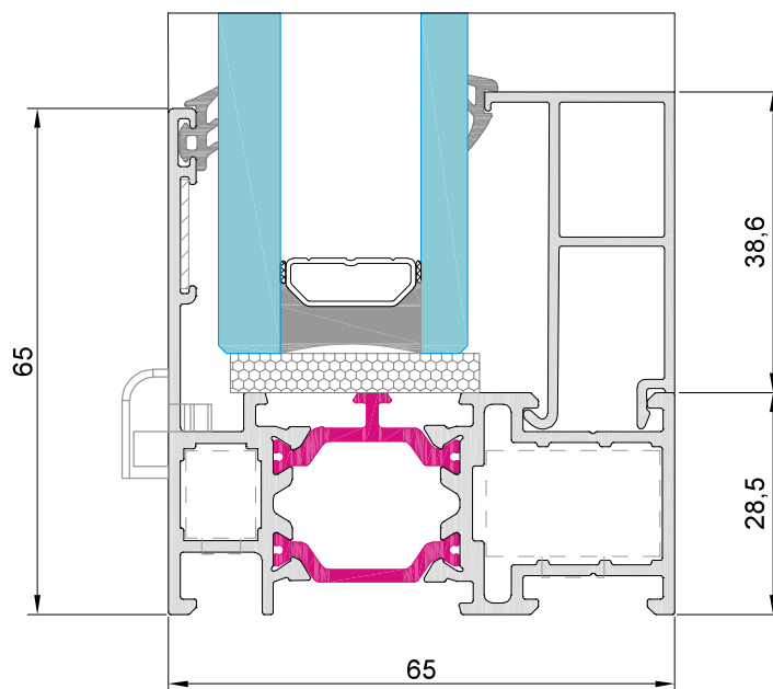
sección 2
