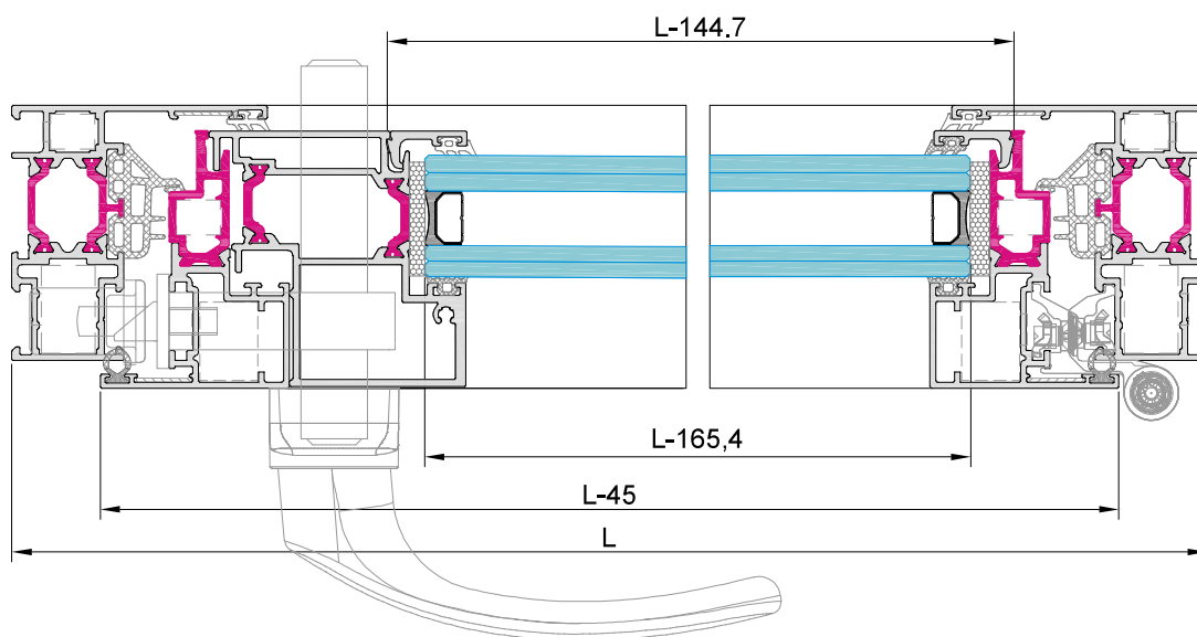
Escala Sección 1:2
