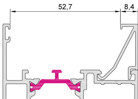
10001 junquillo 8,4 mm
