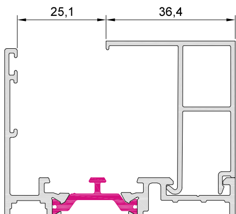
60541 junquillo 36,4 mm
