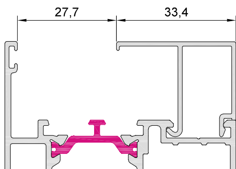
10009 junquillo 33,4 mm
