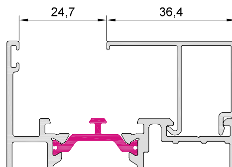
10010 junquillo 36,4 mm
