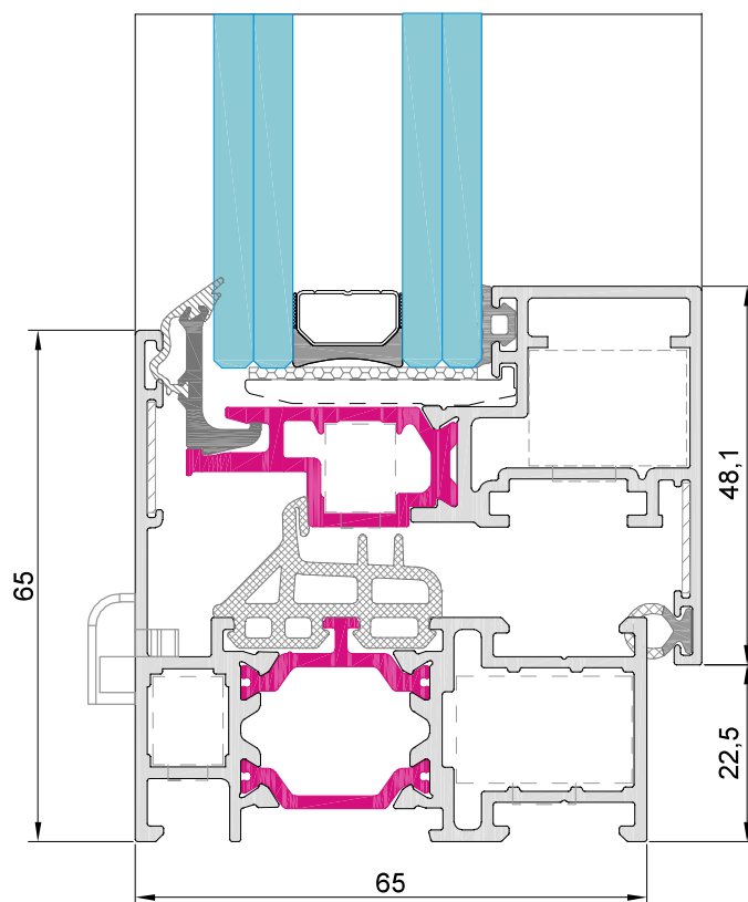
sección 4
