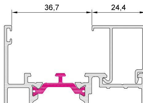
10006 junquillo 24,4 mm
