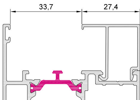
10007 junquillo 27,4 mm
