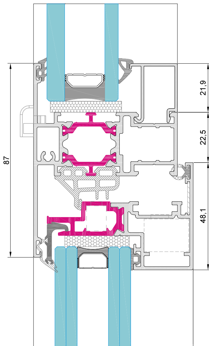
sección 8
