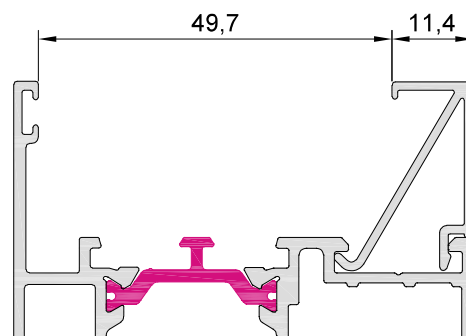
10002 junquillo 11,4 mm
