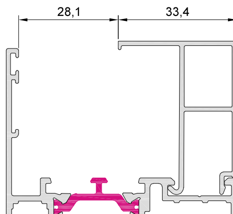
60539 junquillo 33,4 mm
