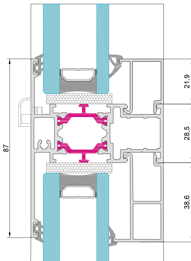
sección 5
