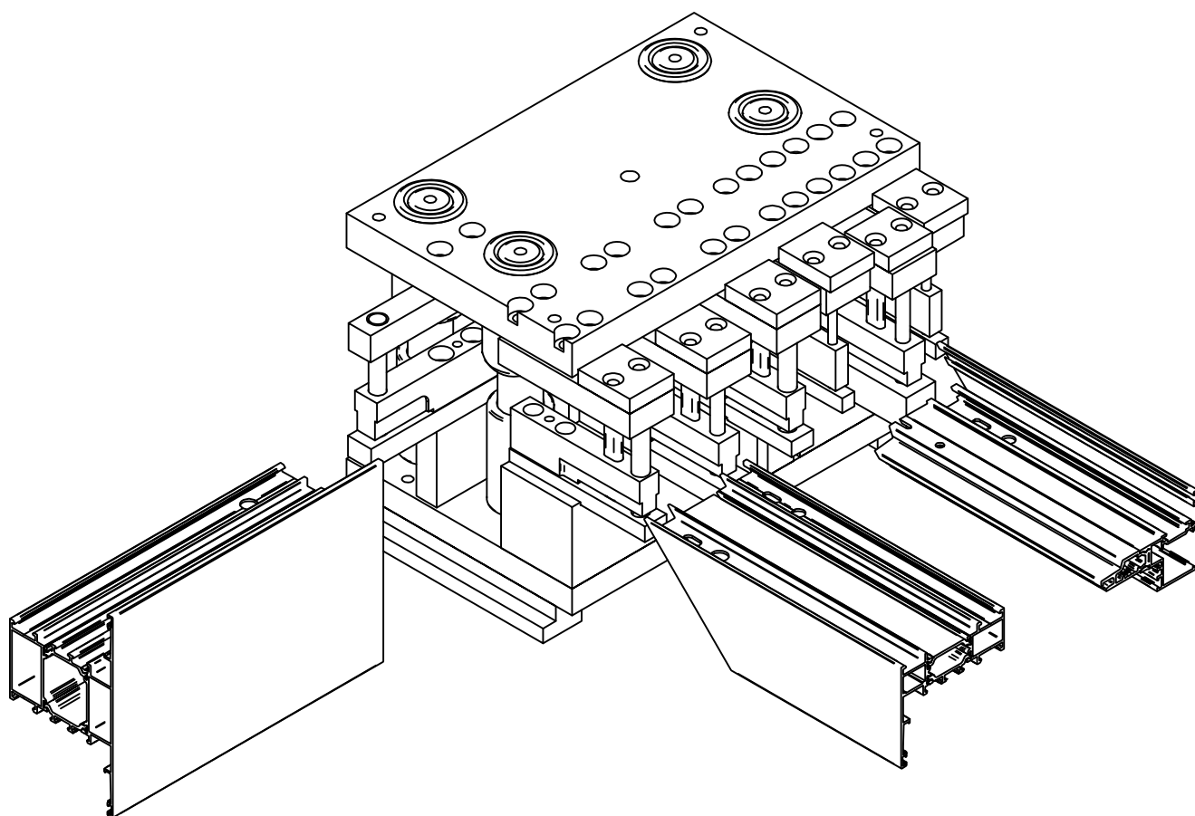
TROQUEL DE MECANIZADO 1503 ESCUADRAS Y UNIÓN T
