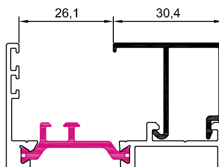
10008 junquillo 30,4 mm
