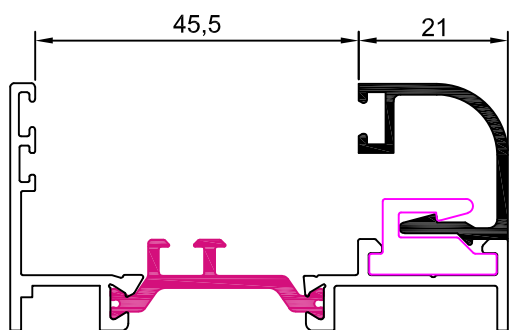
12003 junquillo 21 mm
