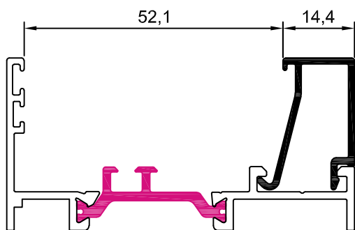
10003 junquillo 14,4 mm
