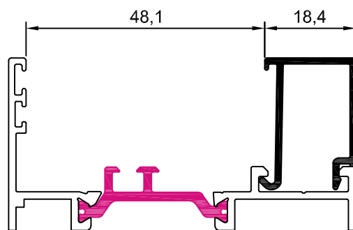
10004 junquillo 18,4 mm
