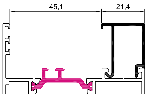
10005 junquillo 21,4 mm
