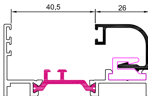
12004 junquillo 26 mm
