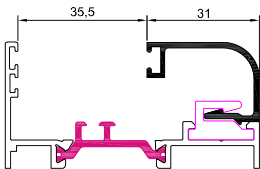
12005 junquillo 31 mm
