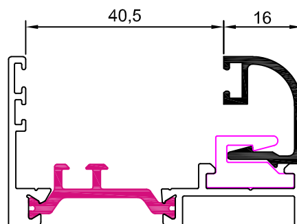
12002 junquillo 16 mm
