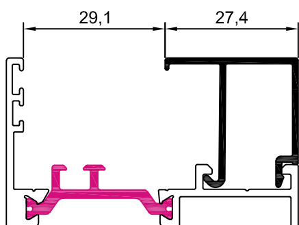
10007 junquillo 27,4 mm
